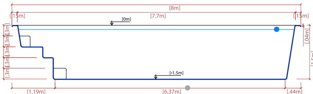
SECTION LONGITUDINALE
