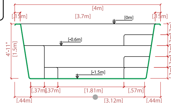
COUPE TRANSVERSALE
