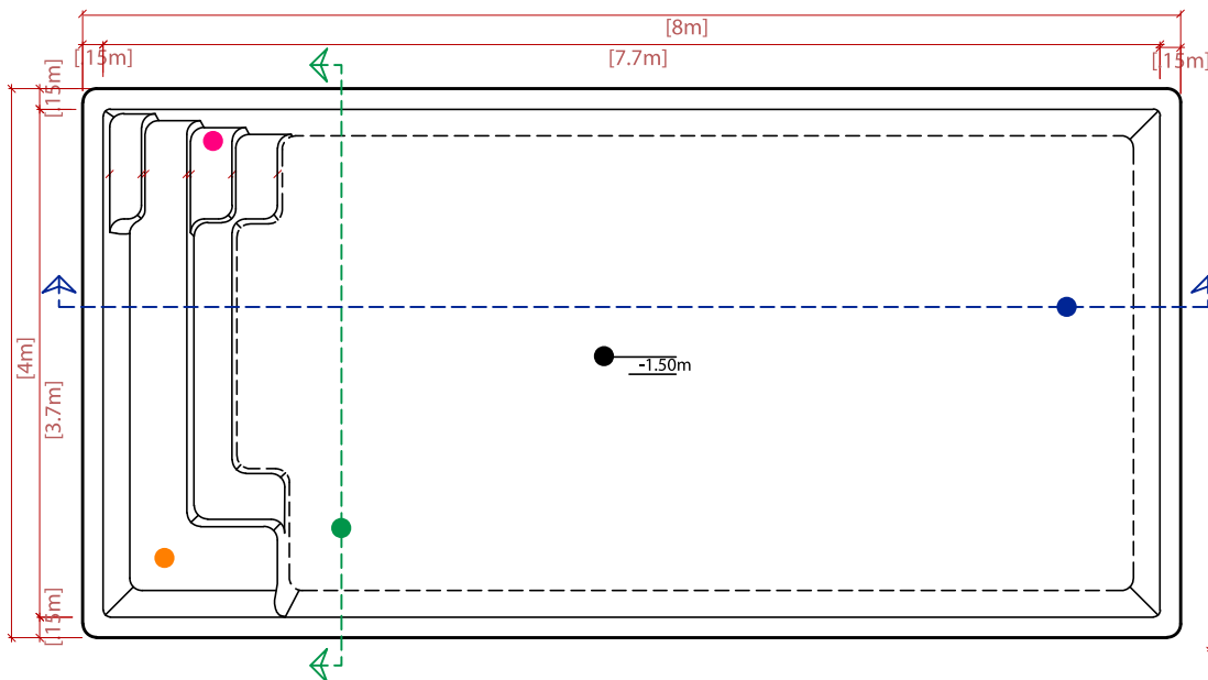
DESSINS TECHNIQUES
