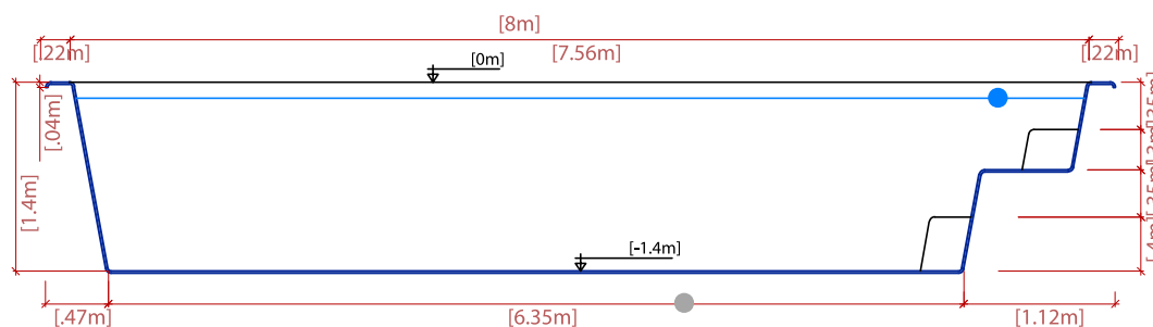
SECTION LONGITUDINALE
