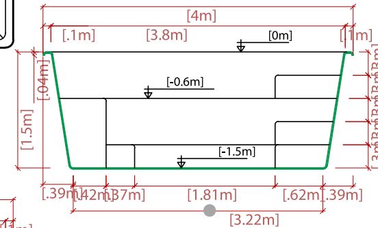
COUPE TRANSVERSALE
