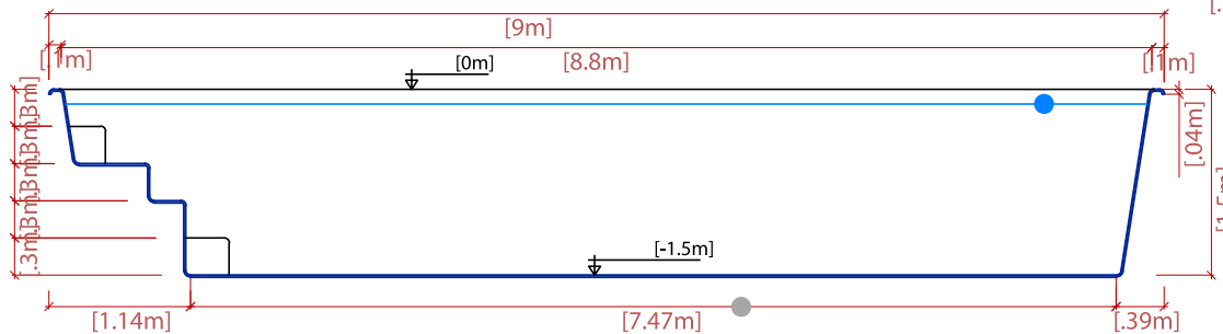
SECTION LONGITUDINALE
