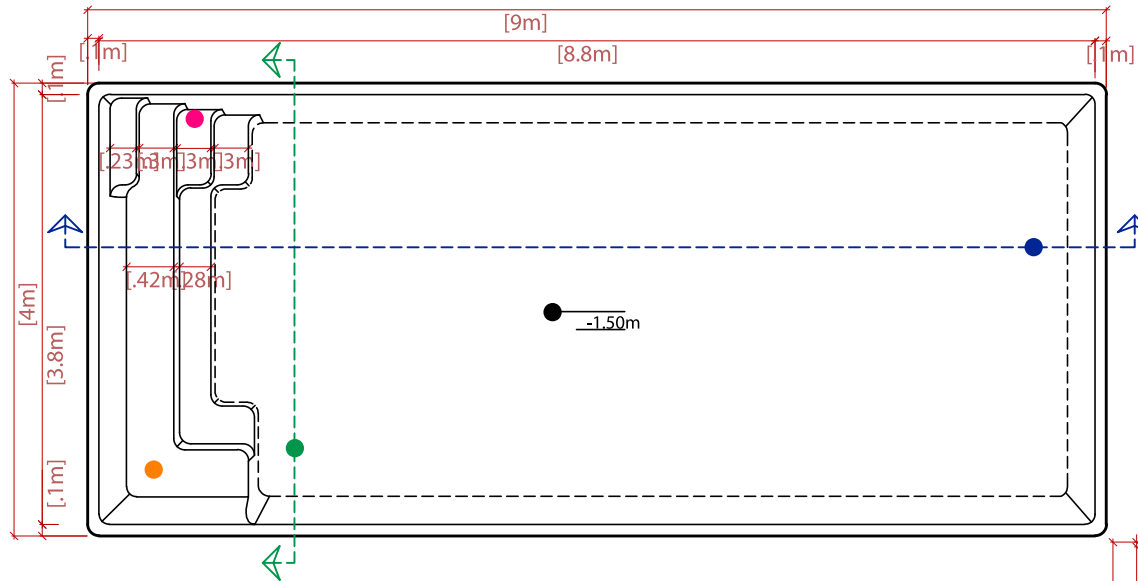
DESSINS TECHNIQUES
