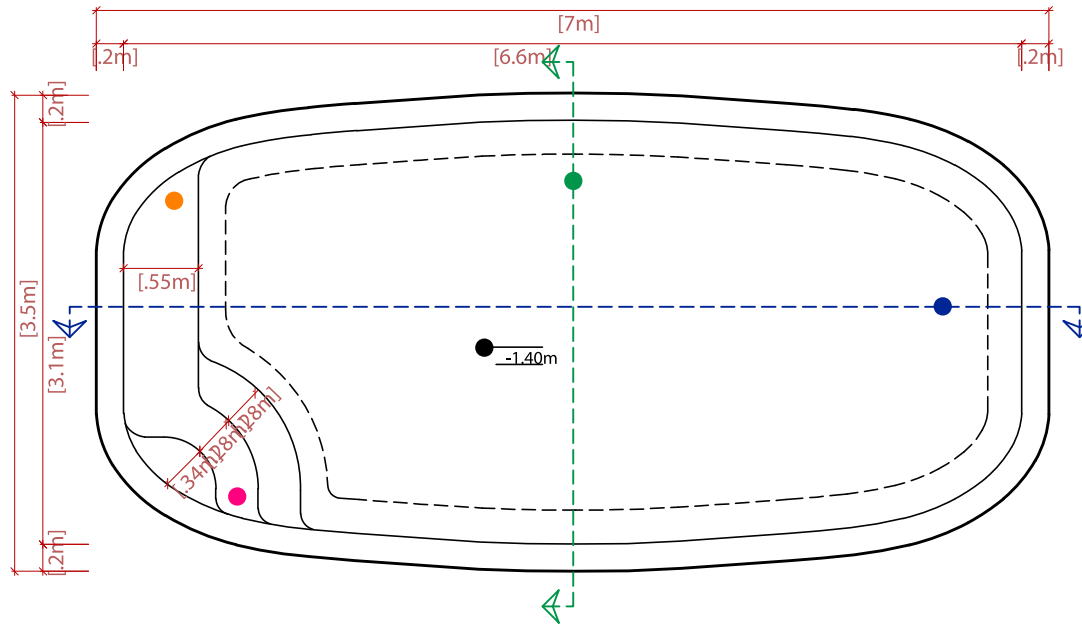
DESSINS TECHNIQUES
