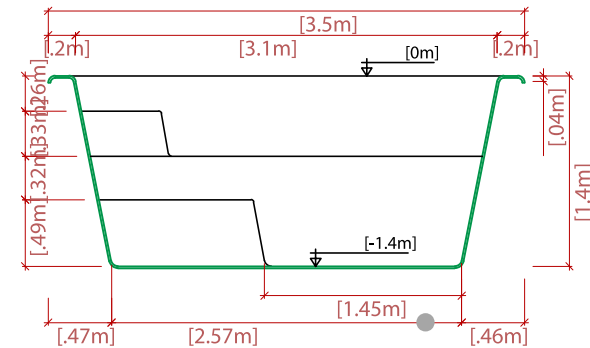
COUPE TRANSVERSALE
