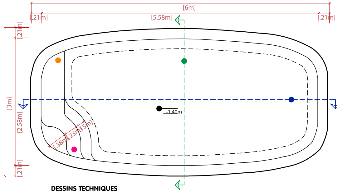
DESSINS TECHNIQUES
