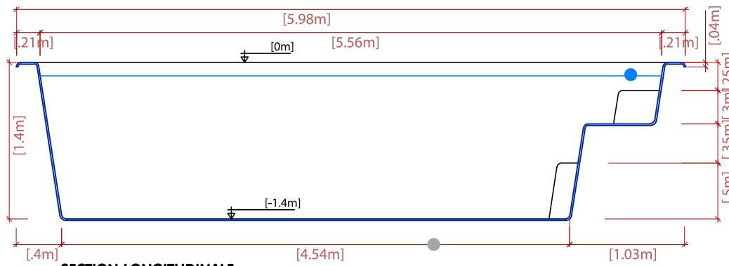
SECTION LONGITUDINALE
