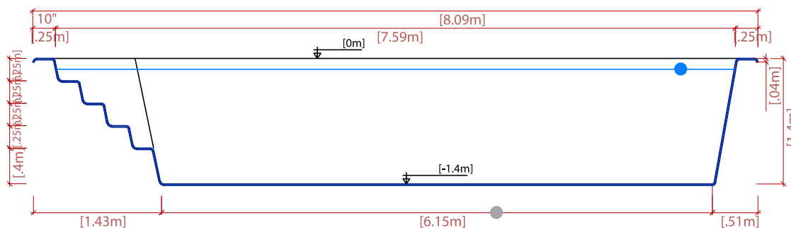
SECTION LONGITUDINALE
