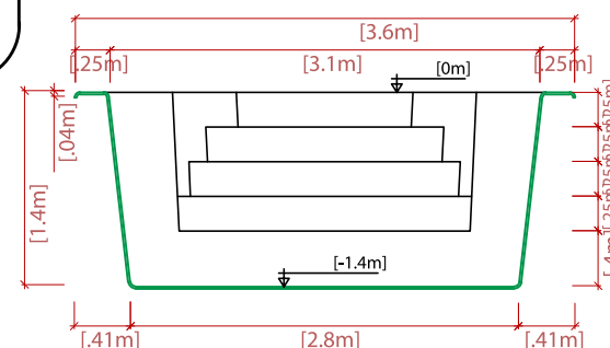
COUPE TRANSVERSALE
